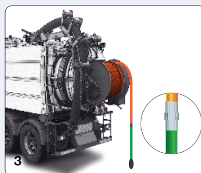
Rubber or thermoplastic "Leader Hose"; to facilitate the operation and to signal the nozzle return. Tubo Leader di gomma o termoplastico che facilita l'operazione di inserimento e segnala l'uscita dell'ugello durante il recupero del tubo.
